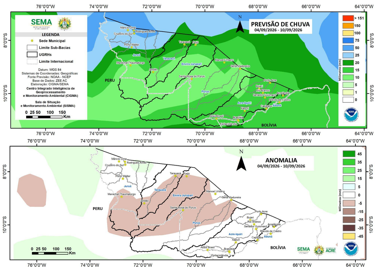
Figura 4: Prognóstico NCEP/GFS.
