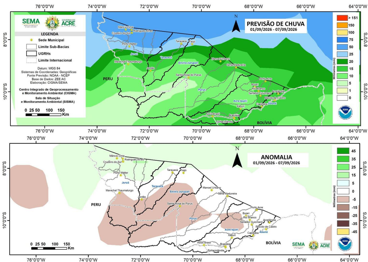
Figura 4: Prognóstico NCEP/GFS.
