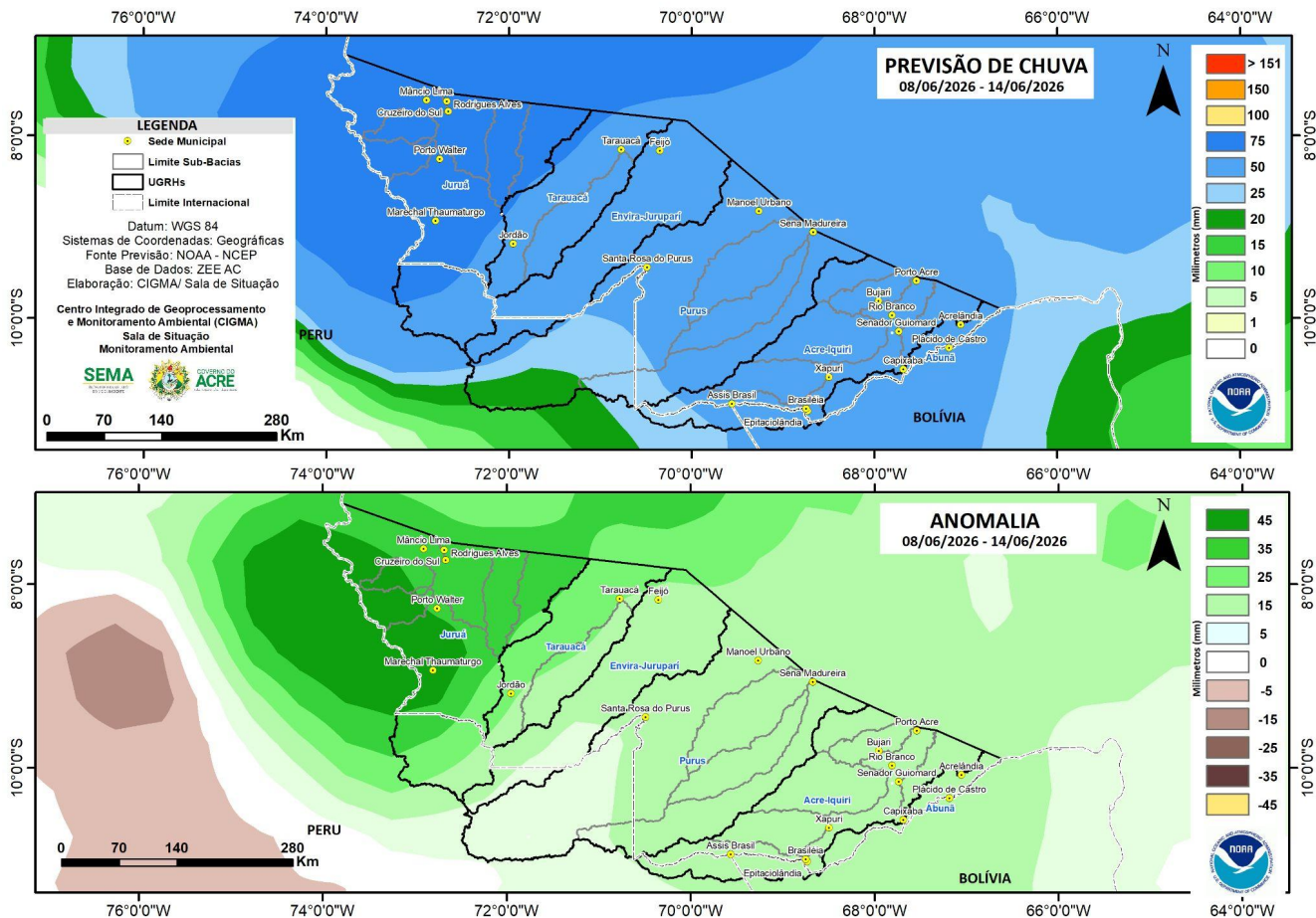
Figura 4: Prognóstico NCEP/GFS.
