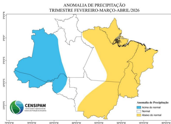
Figura 02 – Prognóstico de anomalias de precipitação para o trimestre Fevereiro, Março e Abril 2026.
