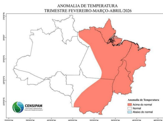
Figura 03 – Prognóstico de anomalias de temperatura para o trimestre Fevereiro, Março e Abril 2026.
