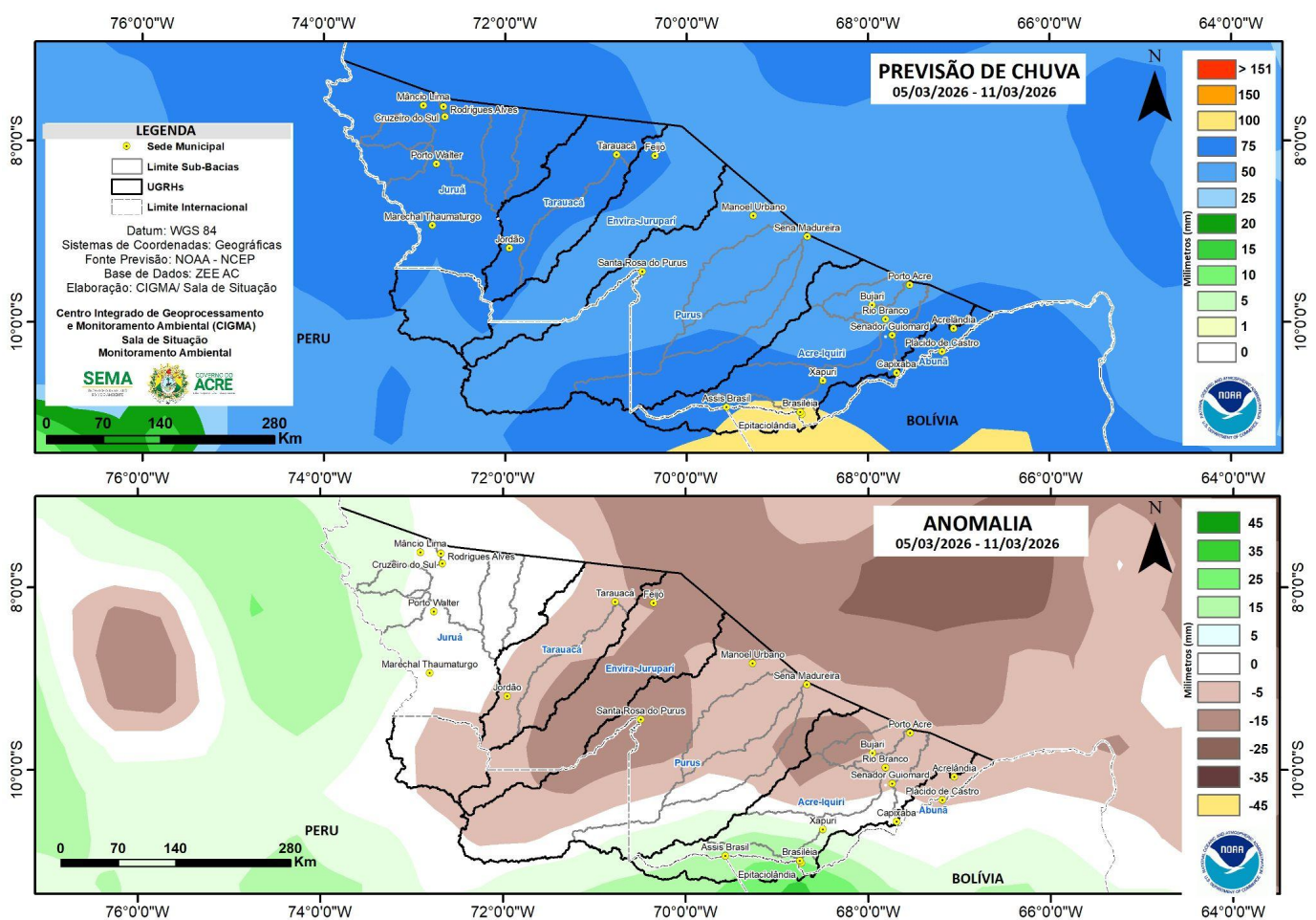
Figura 4: Prognóstico NCEP/GFS.
