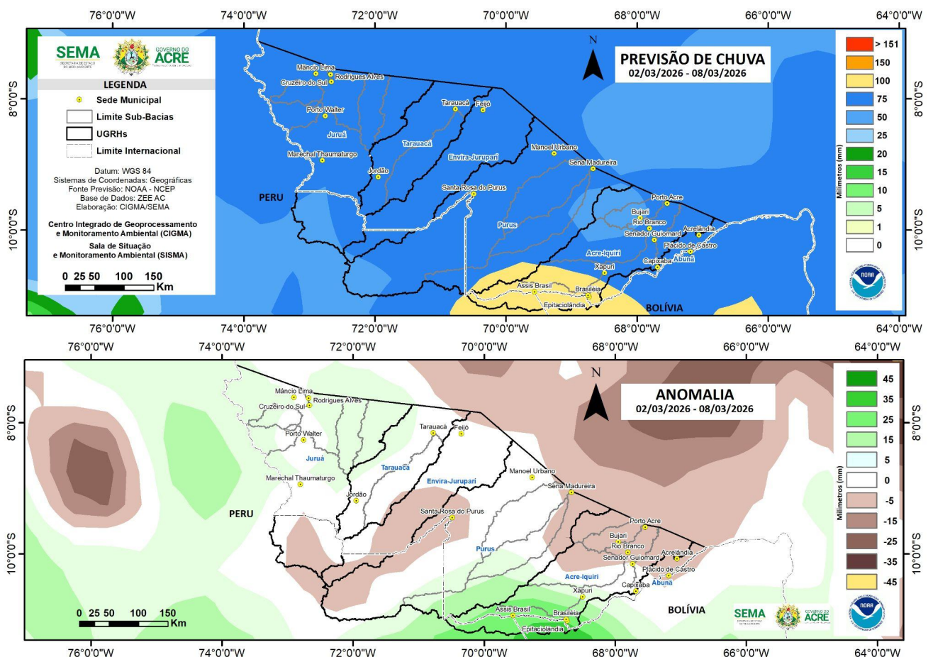
Figura 4: Prognóstico NCEP/GFS.
