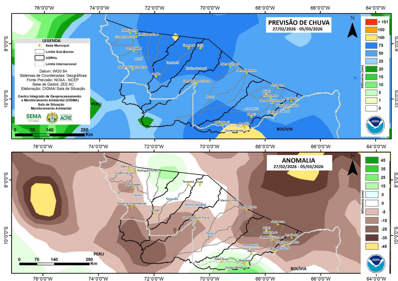
Figura 4: Prognóstico NCEP/GFS.
