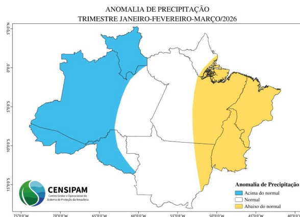
Figura 02 - Prognóstico de anomalias de precipitação para o trimestre Janeiro, Fevereiro e Março .
