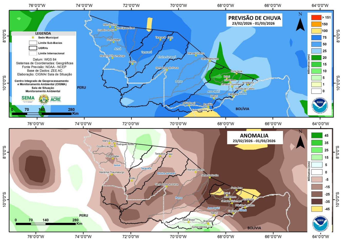
Figura 4: Prognóstico NCEP/GFS.
