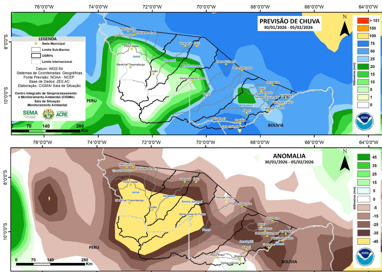
Figura 4: Prognóstico NCEP/GFS.
