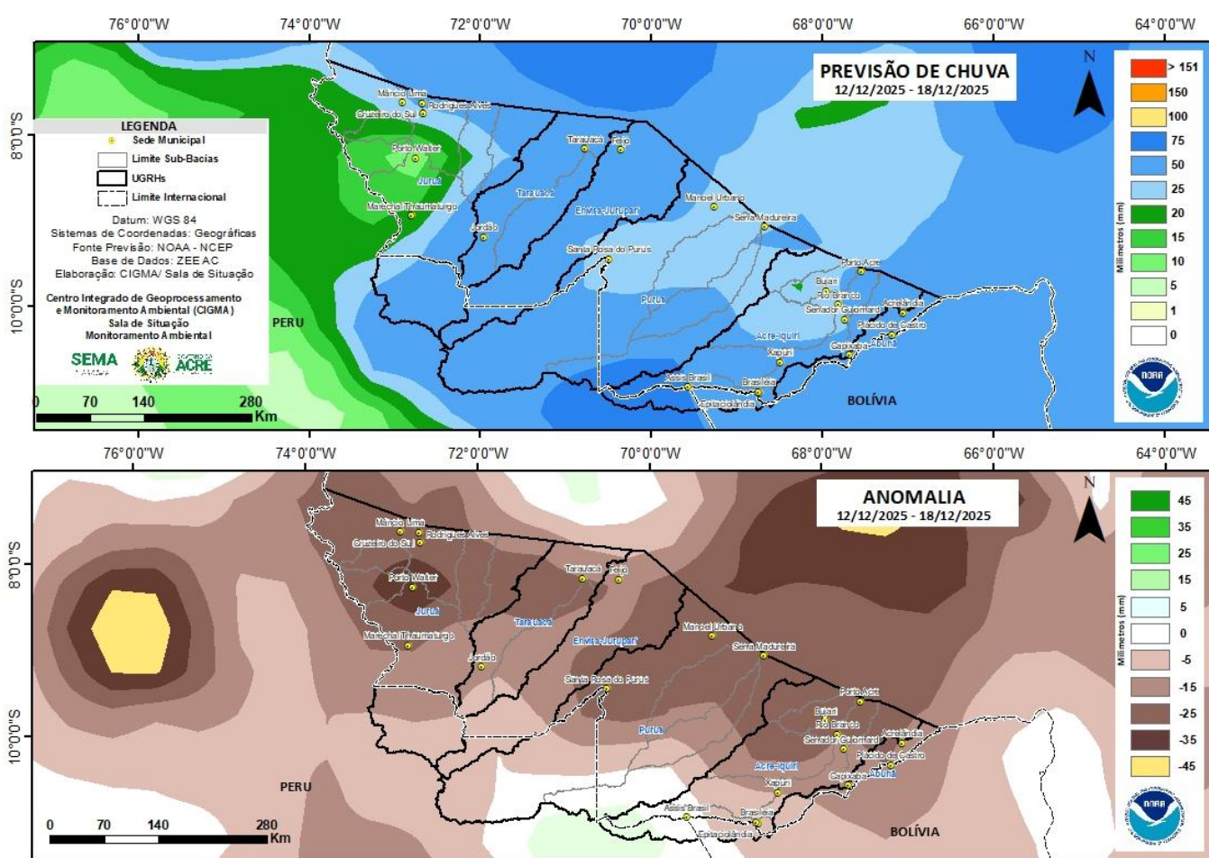
Figura 2: Prognóstico NCEP/GFS.
