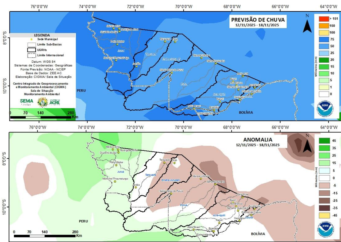
Figura 2: Prognóstico NCEP/GFS.
