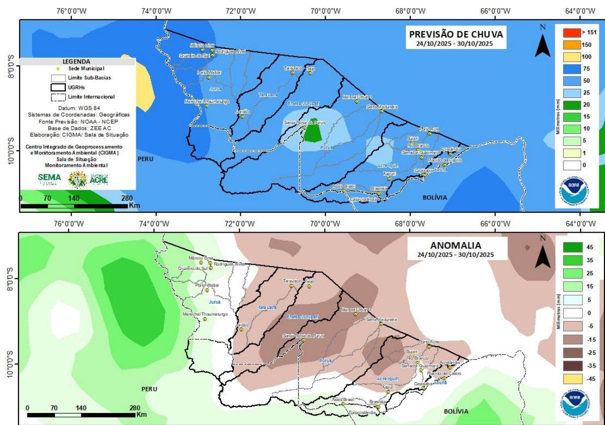
Figura 2: Prognóstico NCEP/GFS.
