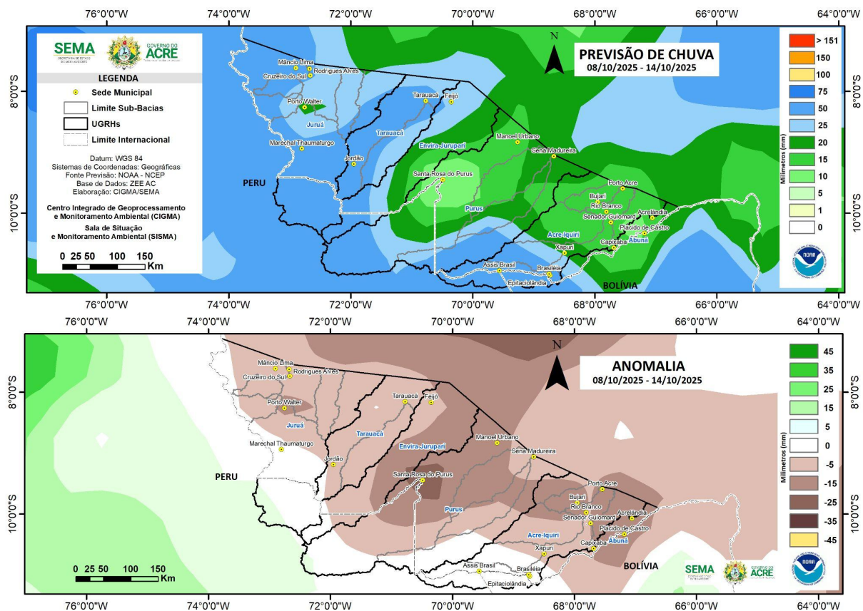
Figura 2: Prognóstico NCEP/GFS.
