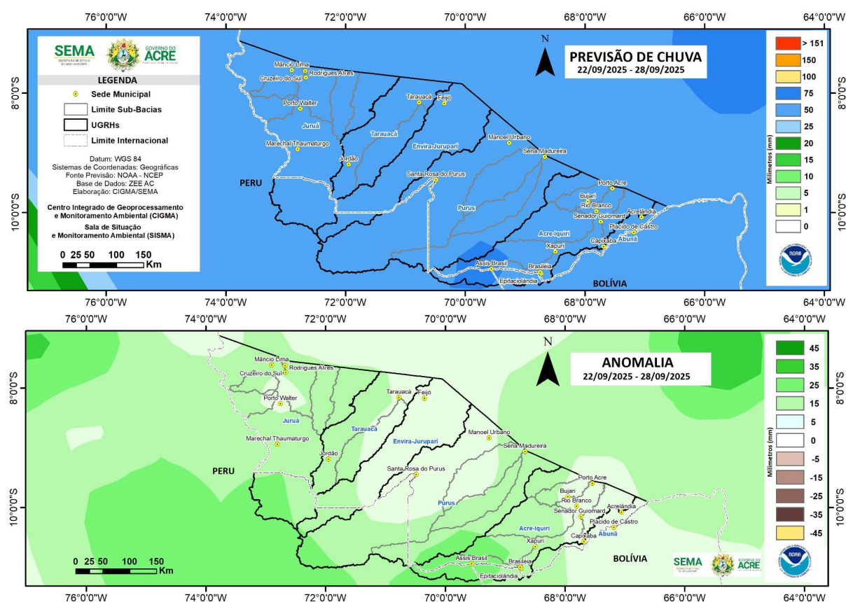
Figura 2: Prognóstico NCEP/GFS.
