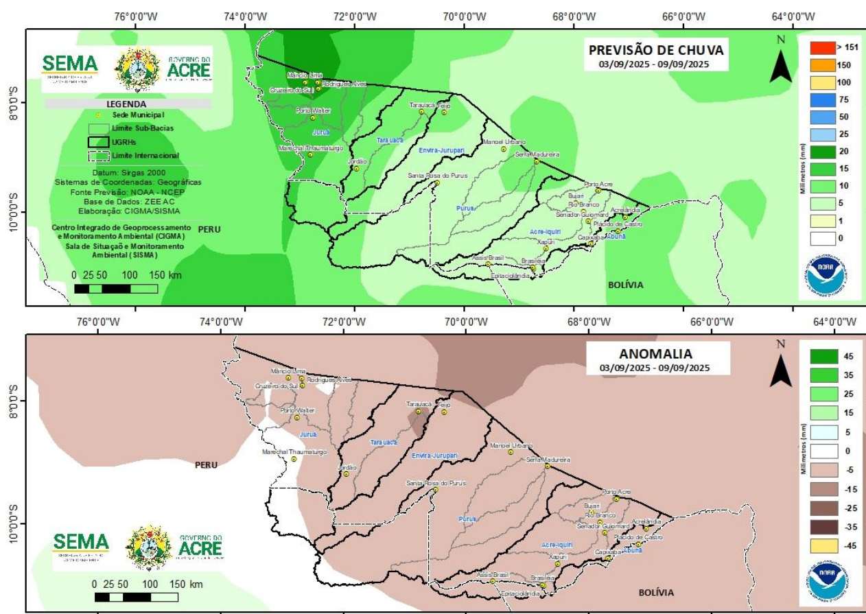
Figura 2: Prognóstico NCEP/GFS.
