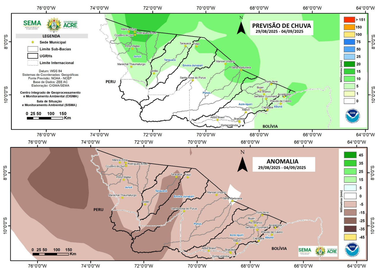
Figura 2: Prognóstico NCEP/GFS.
