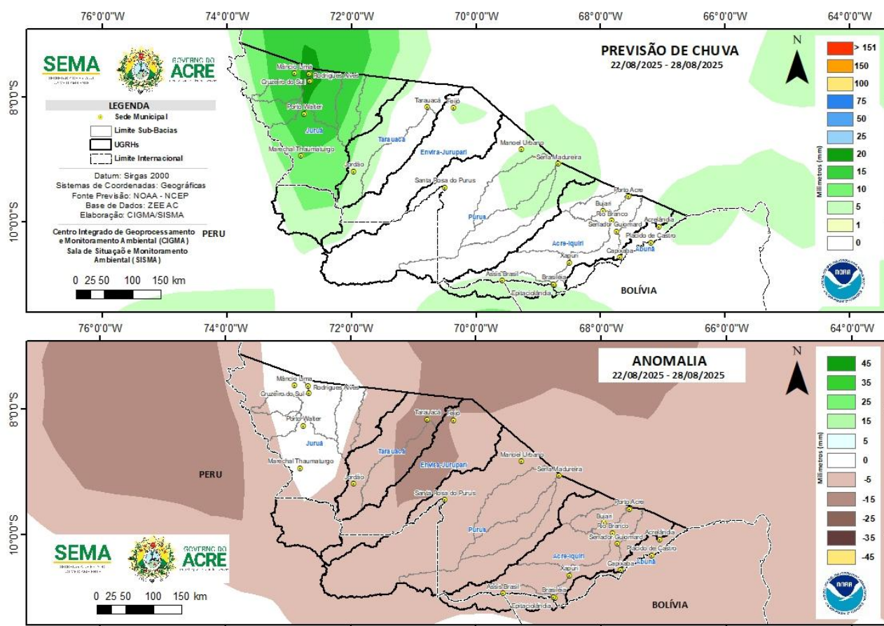
Figura 2: Prognóstico NCEP/GFS.
