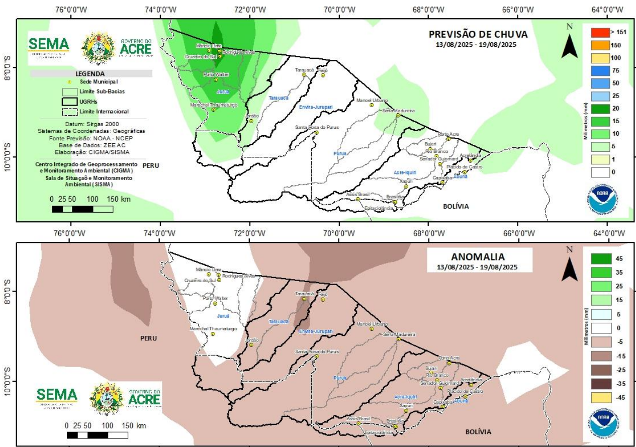
Figura 2: Prognóstico NCEP/GFS.
