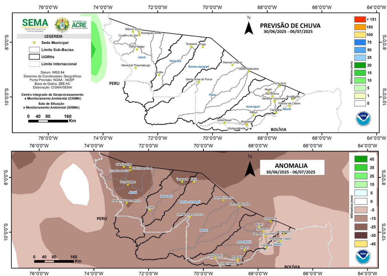
Figura 2: Prognóstico NCEP/GFS
