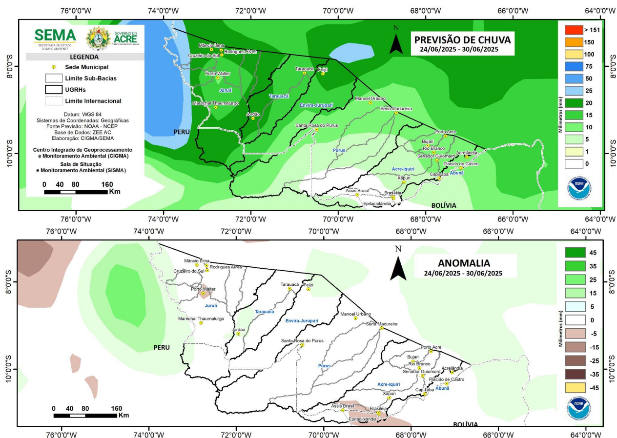
Figura 2: Prognóstico NCEP/GFS
