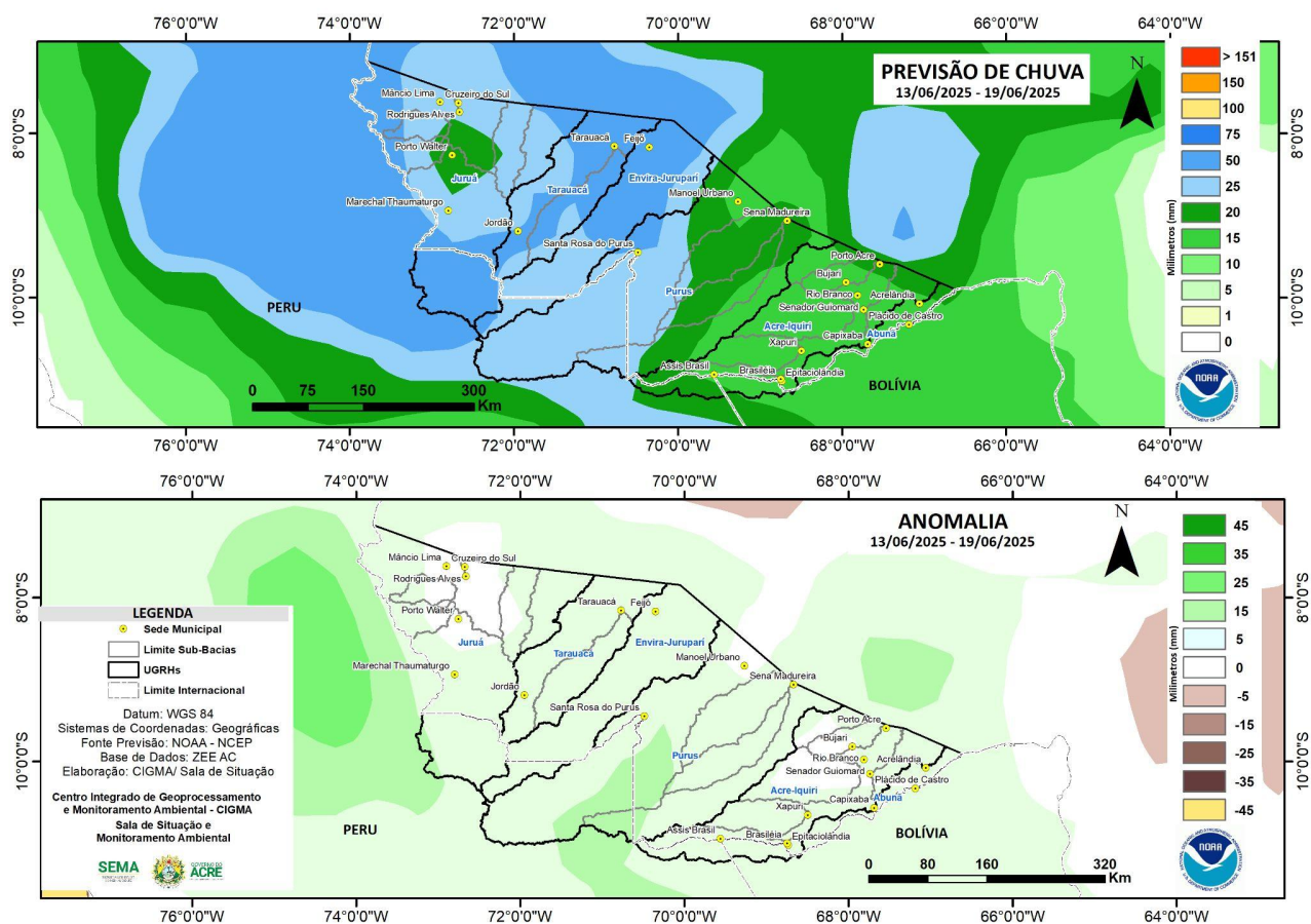
Figura 2: Prognóstico NCEP/GFS
