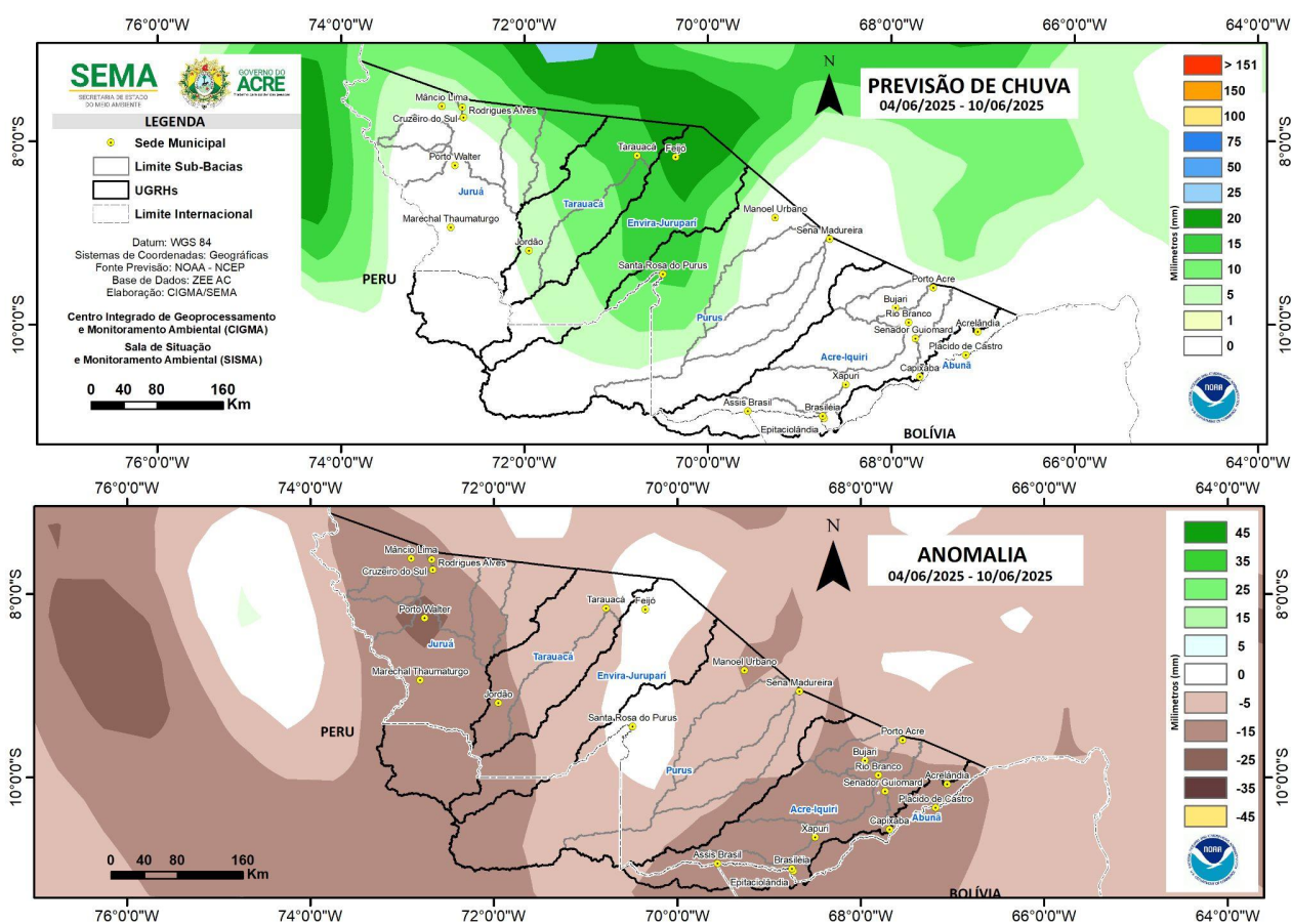
Figura 2: Prognóstico NCEP/GFS
