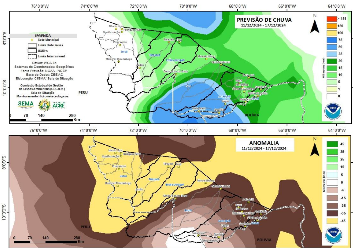
Figura 2: Prognóstico NCEP/GFS
