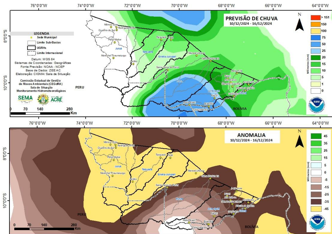
Figura 2: Prognóstico NCEP/GFS
