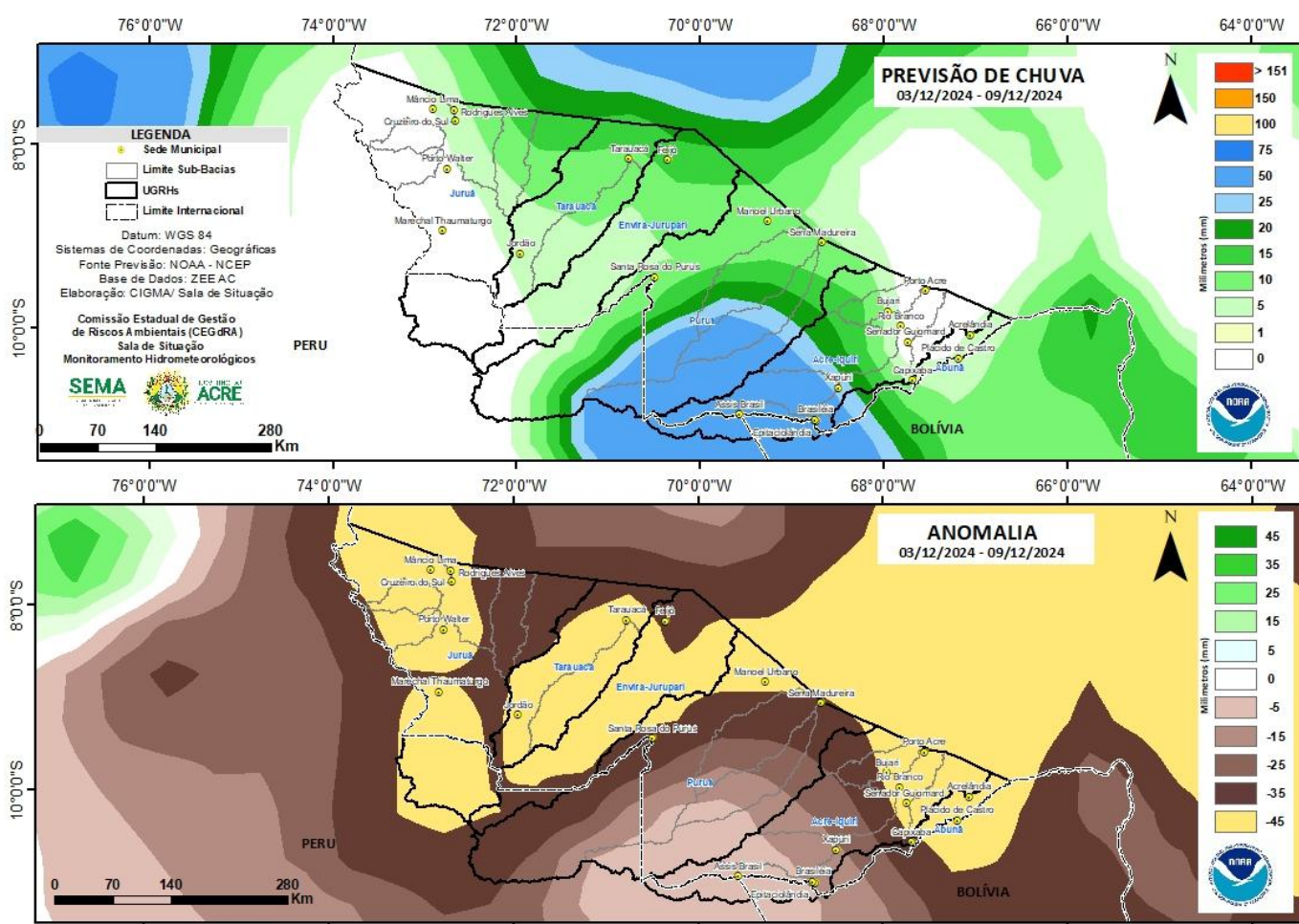
Figura 2: Prognóstico NCEP/GFS
