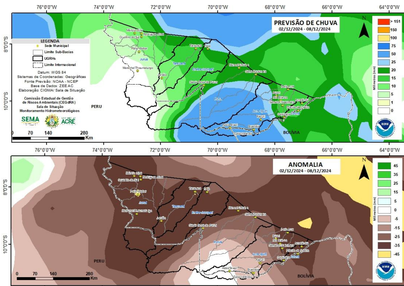
Figura 2: Prognóstico NCEP/GFS
