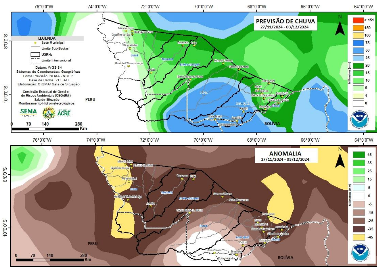
Figura 2: Prognóstico NCEP/GFS
