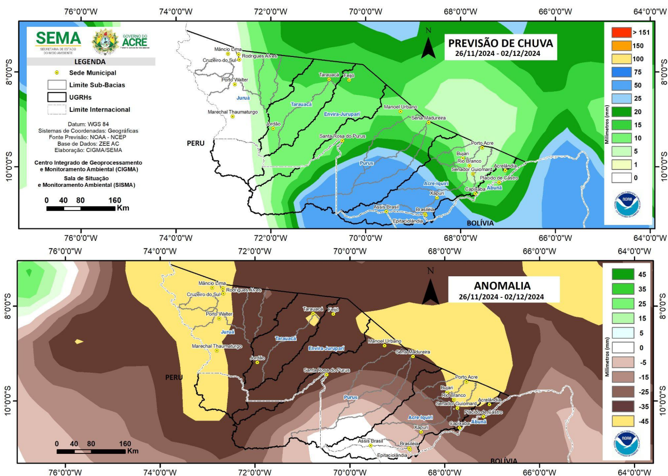
Figura 2: Prognóstico NCEP/GFS
