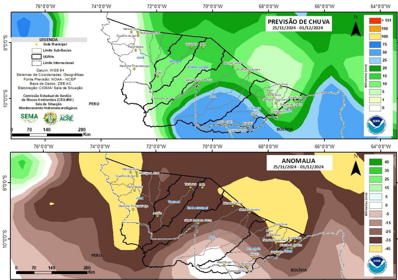
Figura 2: Prognóstico NCEP/GFS
