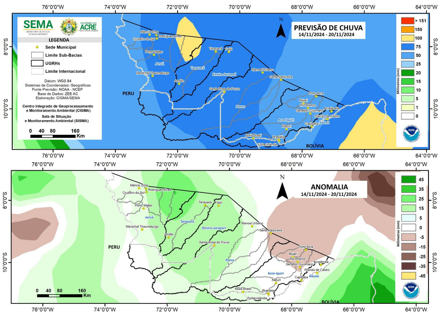
Figura 2: Prognóstico NCEP/GFS
