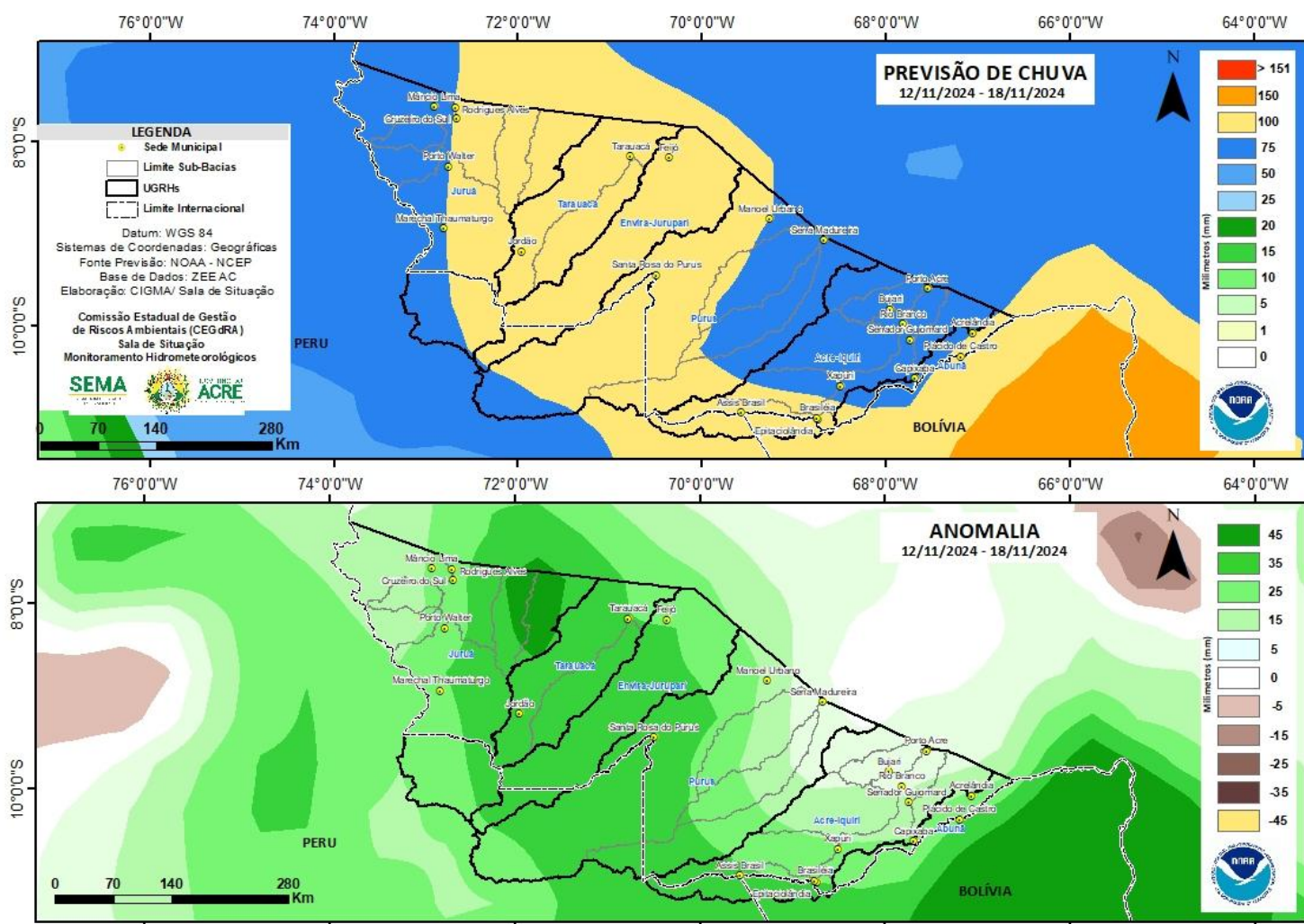
Figura 2: Prognóstico NCEP/GFS
