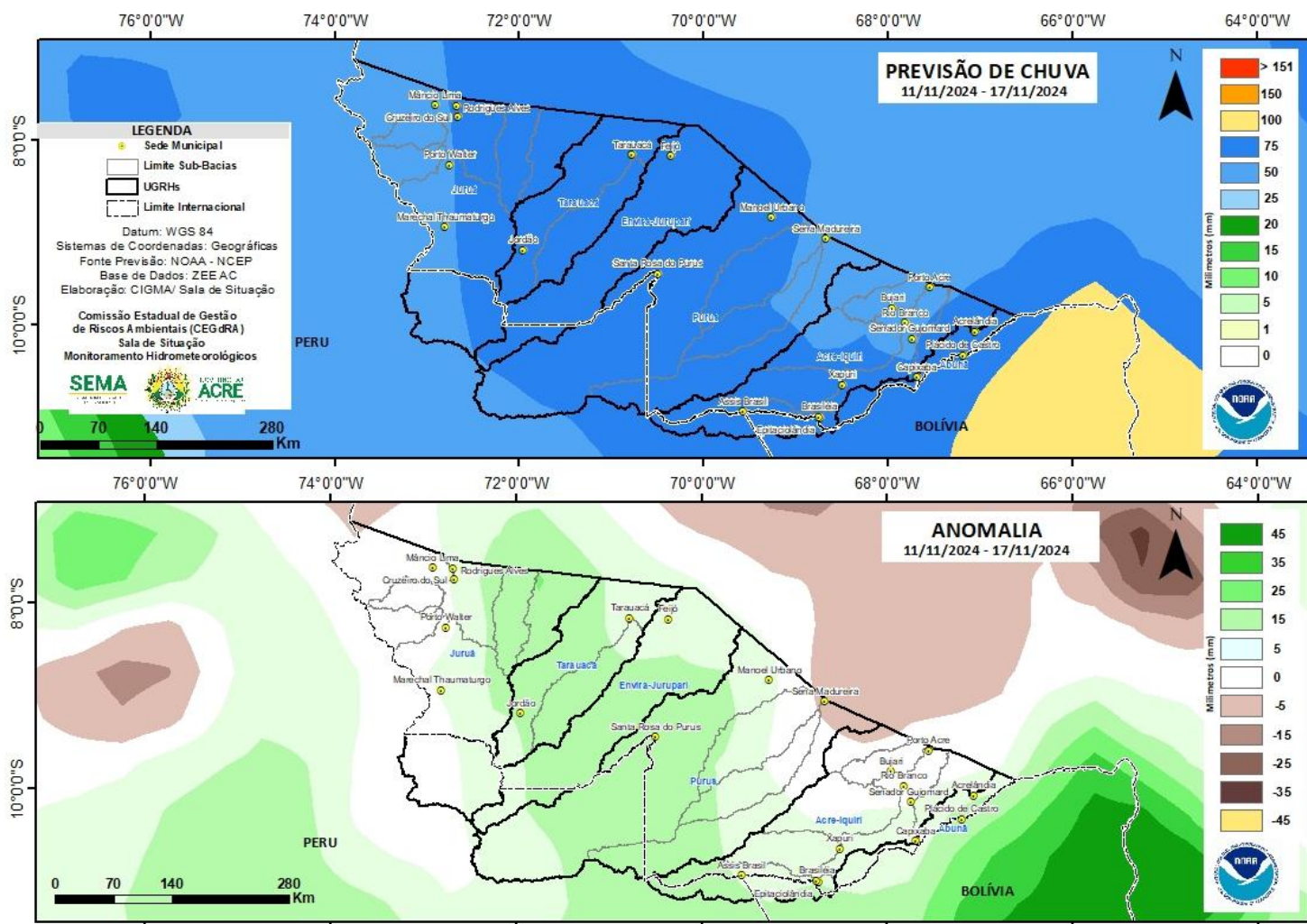
Figura 2: Prognóstico NCEP/GFS
