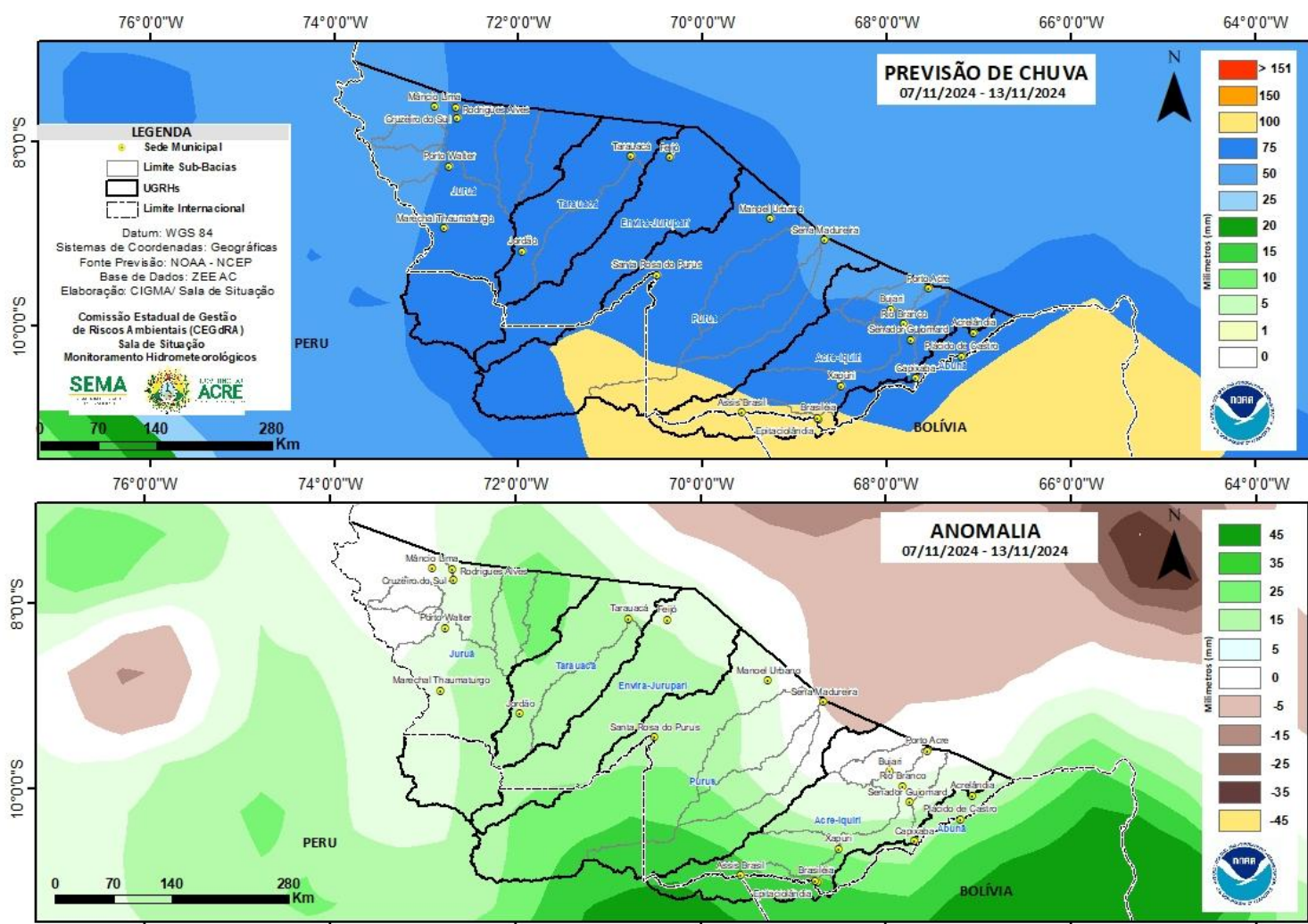
Figura 2: Prognóstico NCEP/GFS
