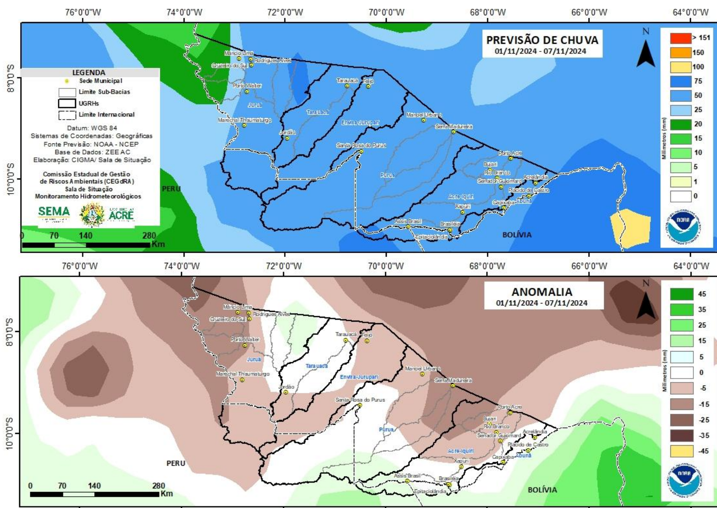
Figura 2: Prognóstico NCEP/GFS
