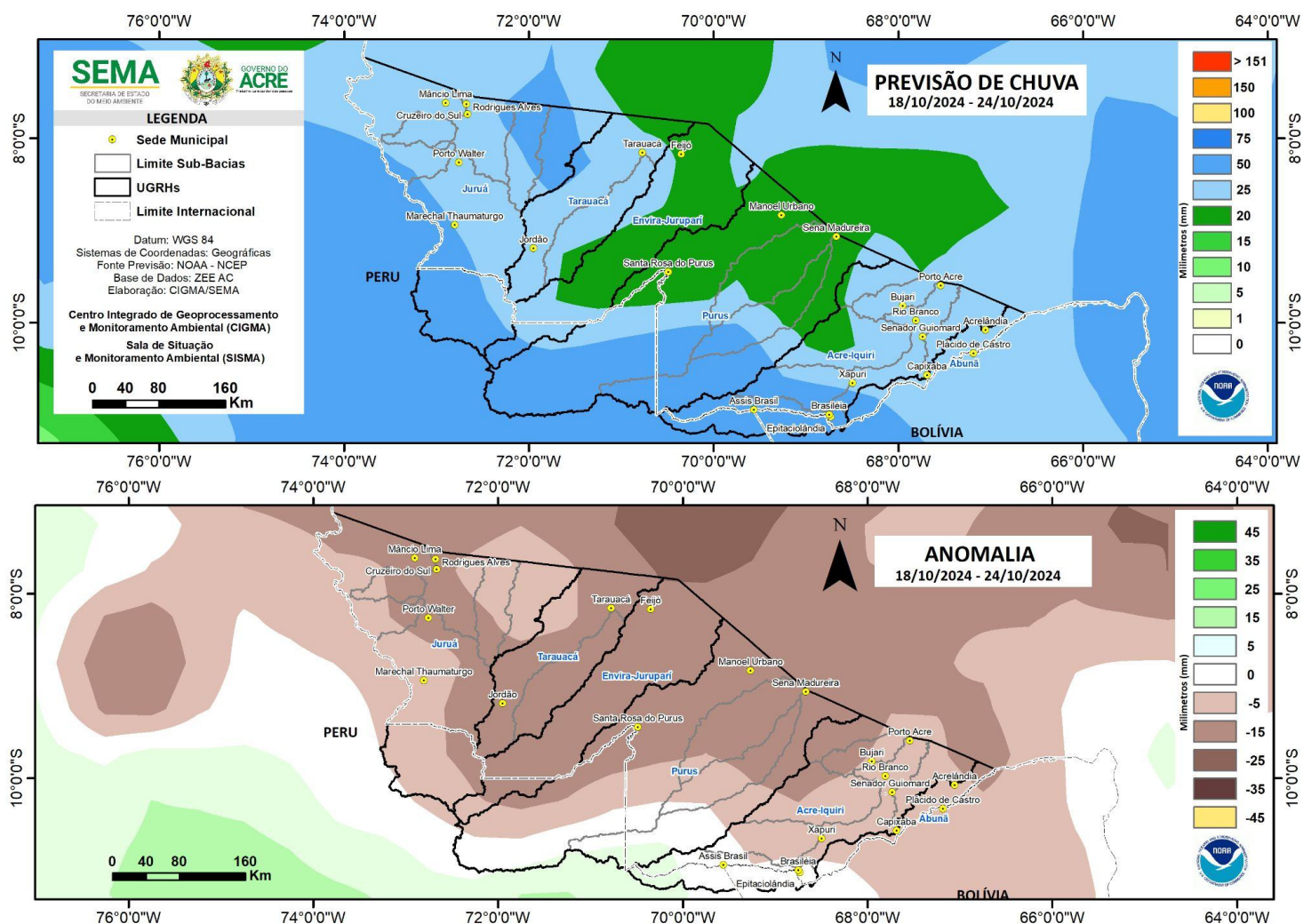
Figura 2: Prognóstico NCEP/GFS
