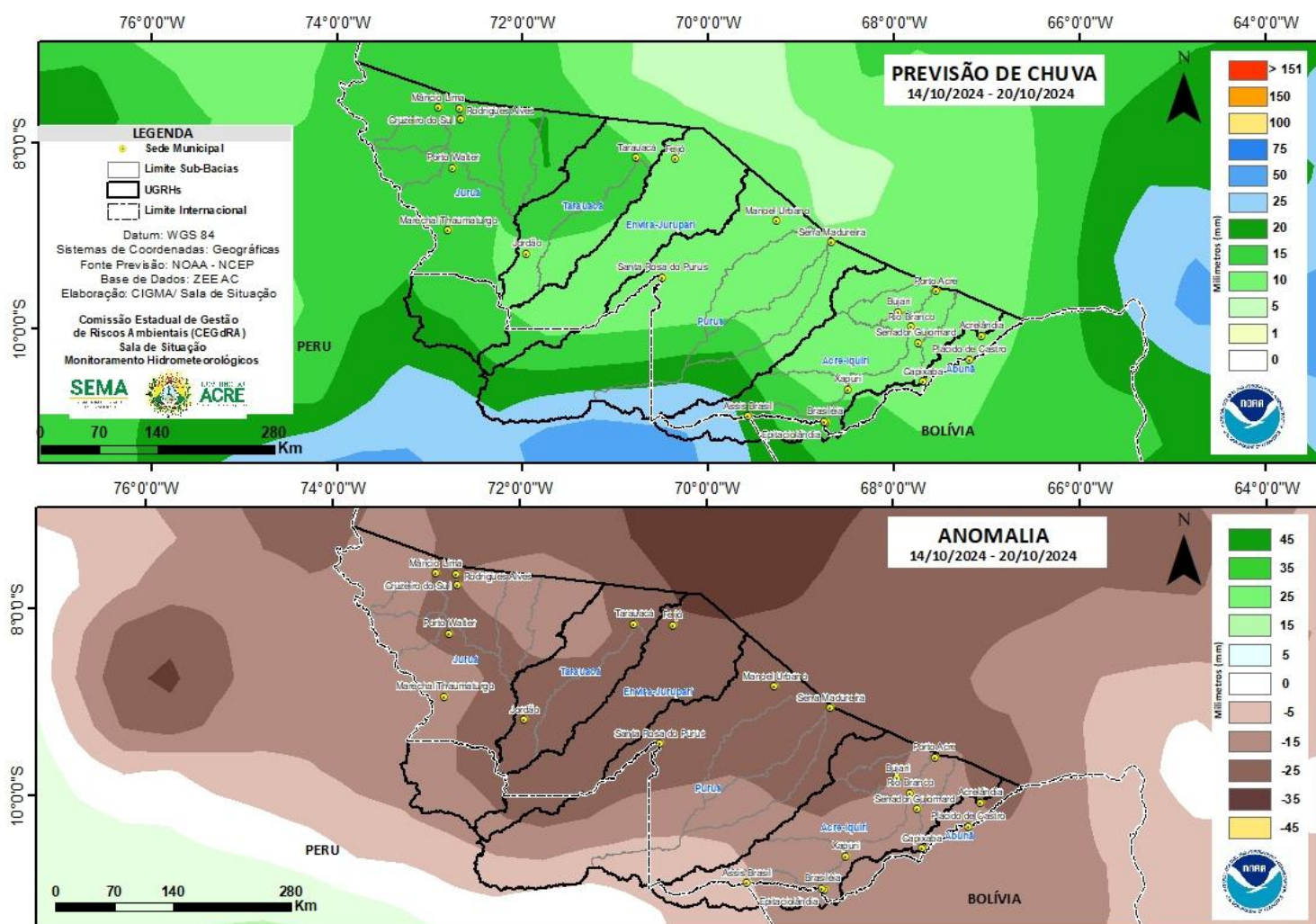
Figura 2: Prognóstico NCEP/GFS
