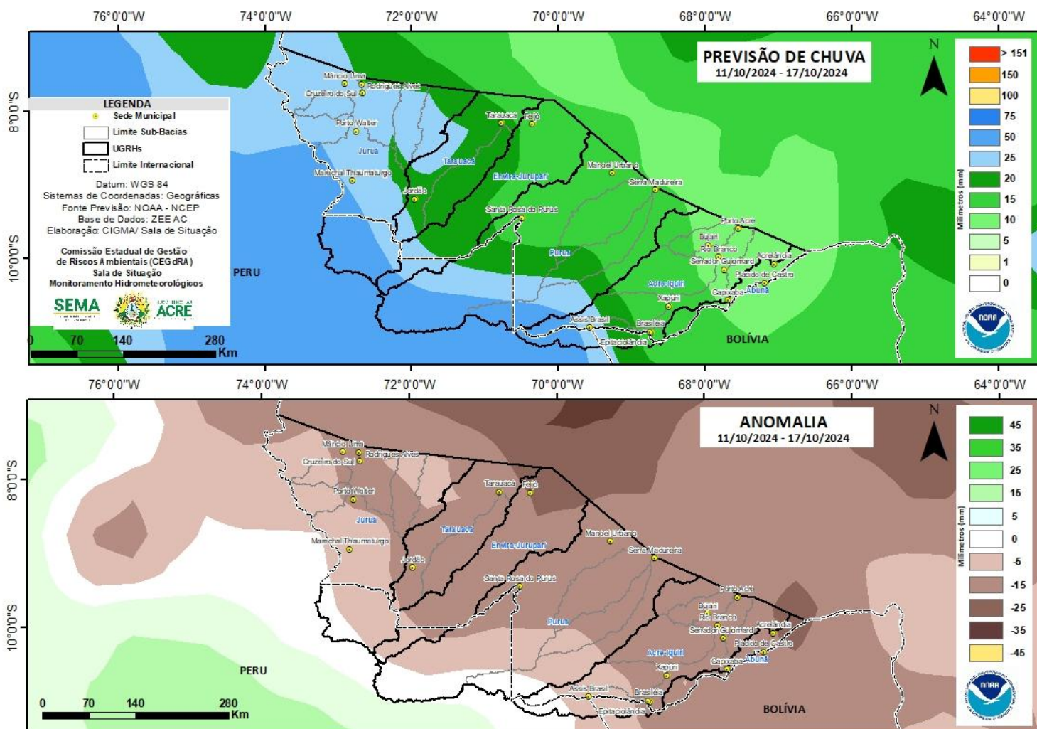
Figura 2: Prognóstico NCEP/GFS
