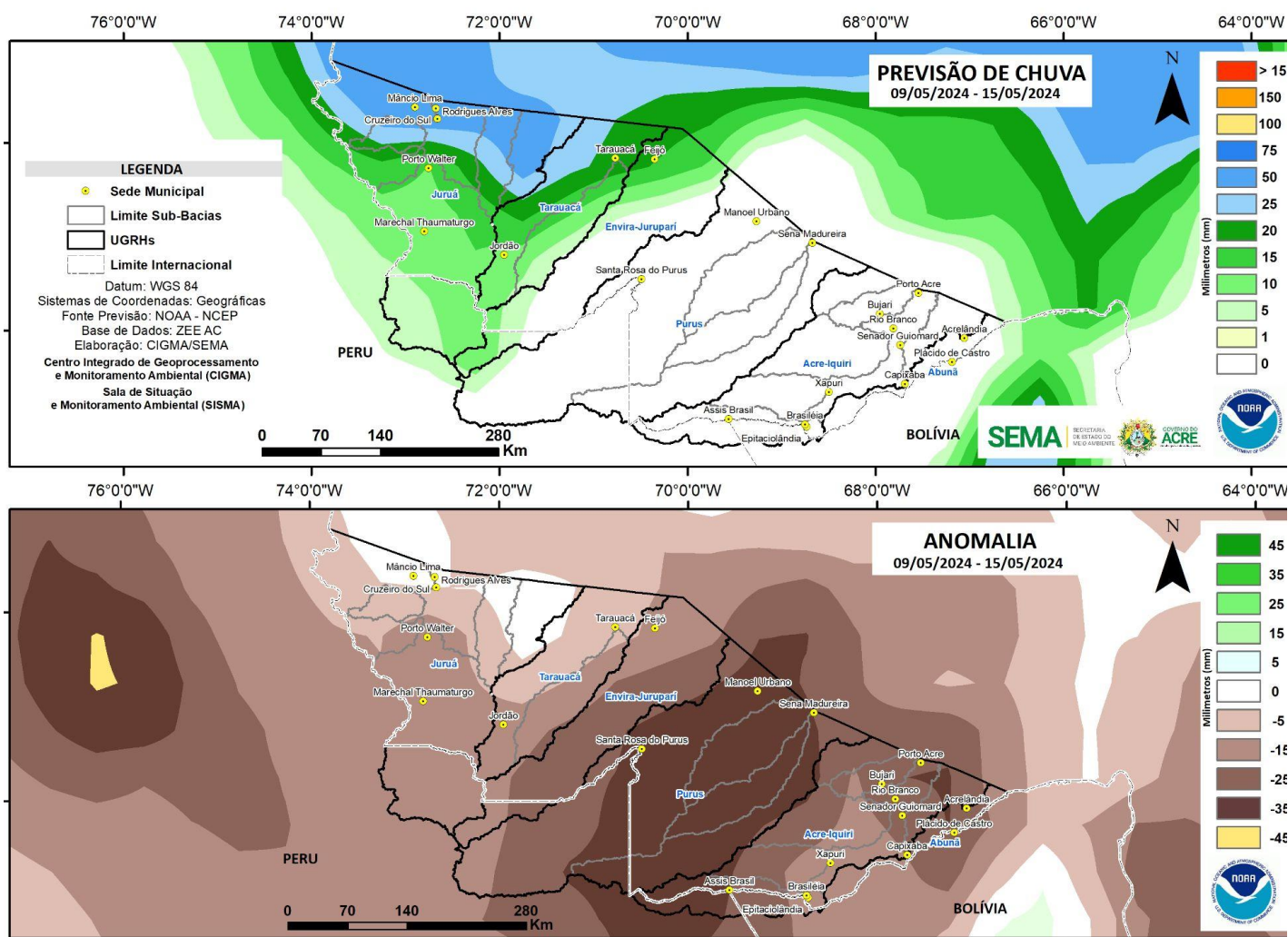
Figura 2: Prognóstico NCEP-GFS
