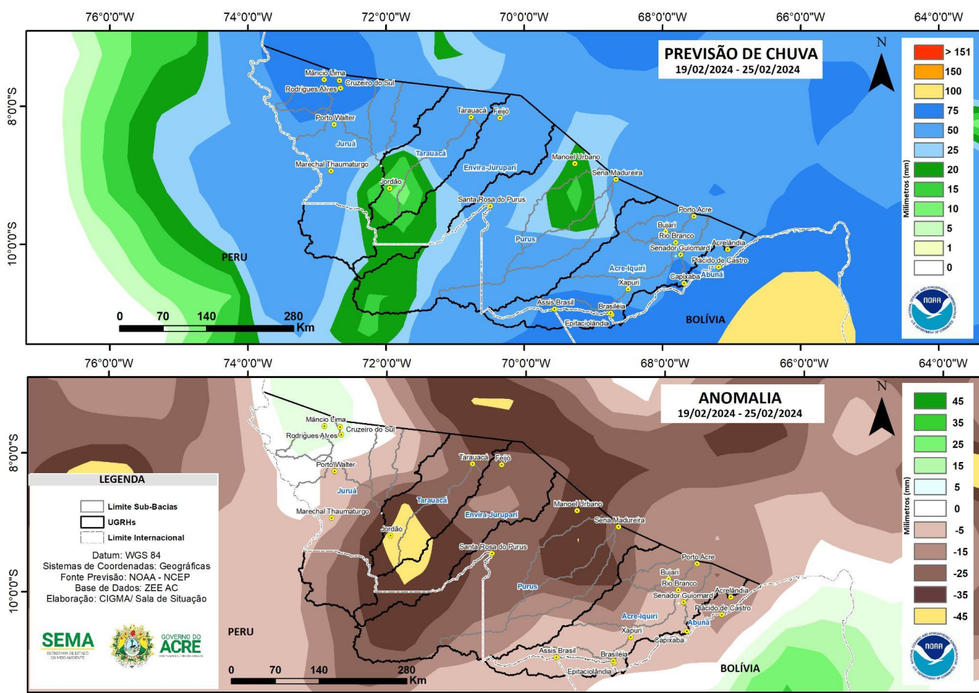
Figura 2: Prognóstico NCEP-GFS
