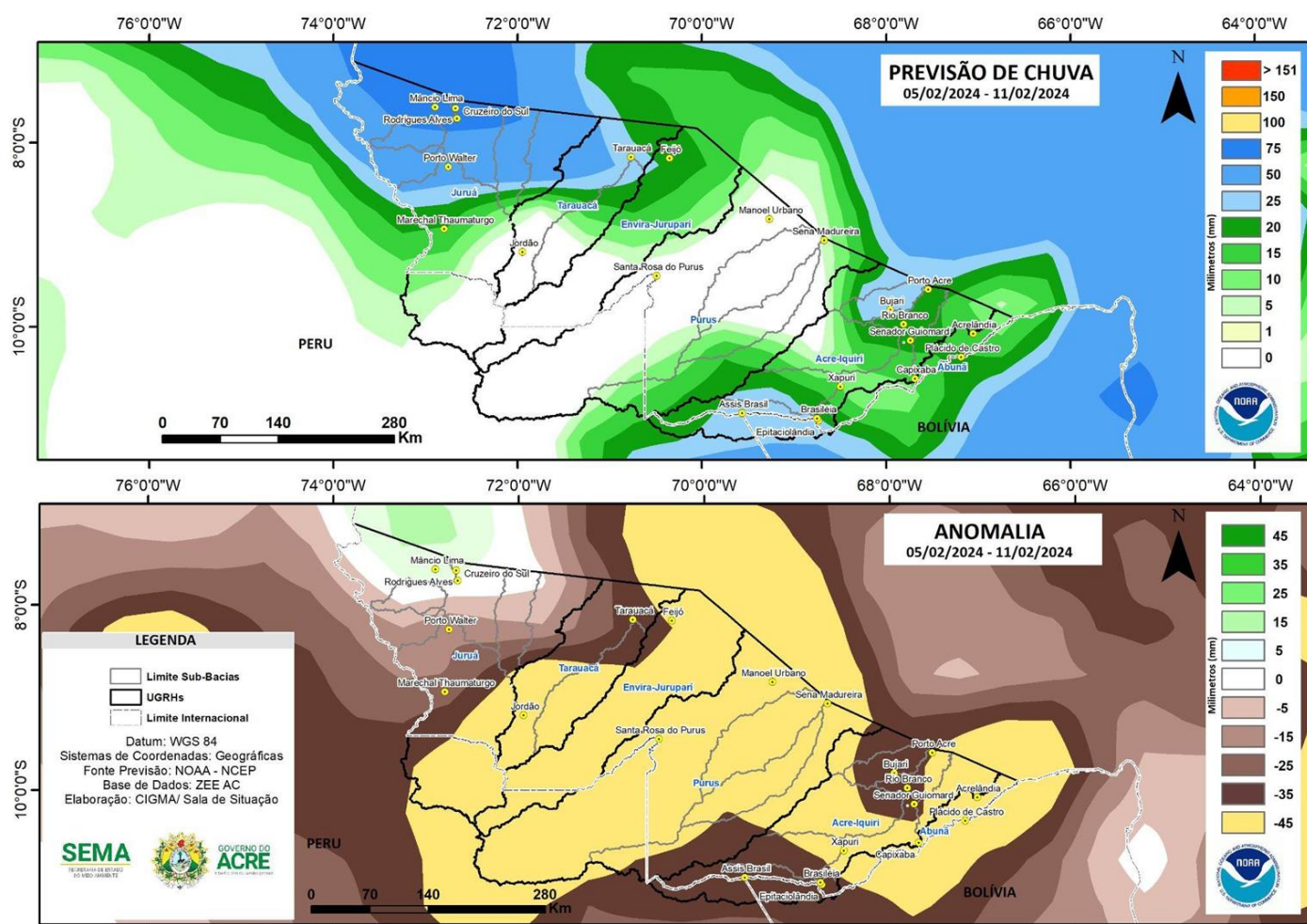
Figura 2: Prognóstico NCEP-GFS
