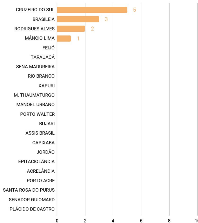
Acumulado de Focos (01/01/2024 a 18/02/2024) Satélite de Referência (AQUA Tarde)
