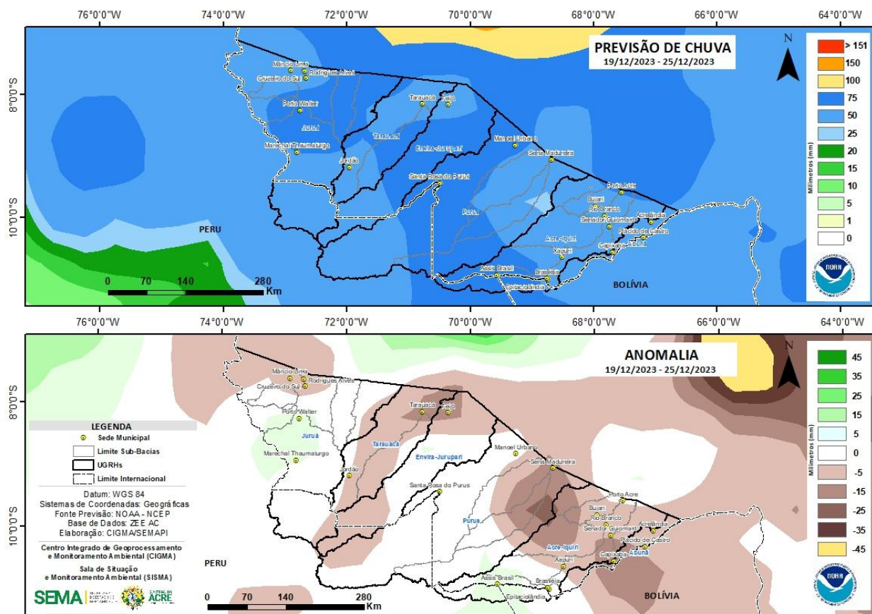
Figura 2: Prognóstico NCEP-GFS
