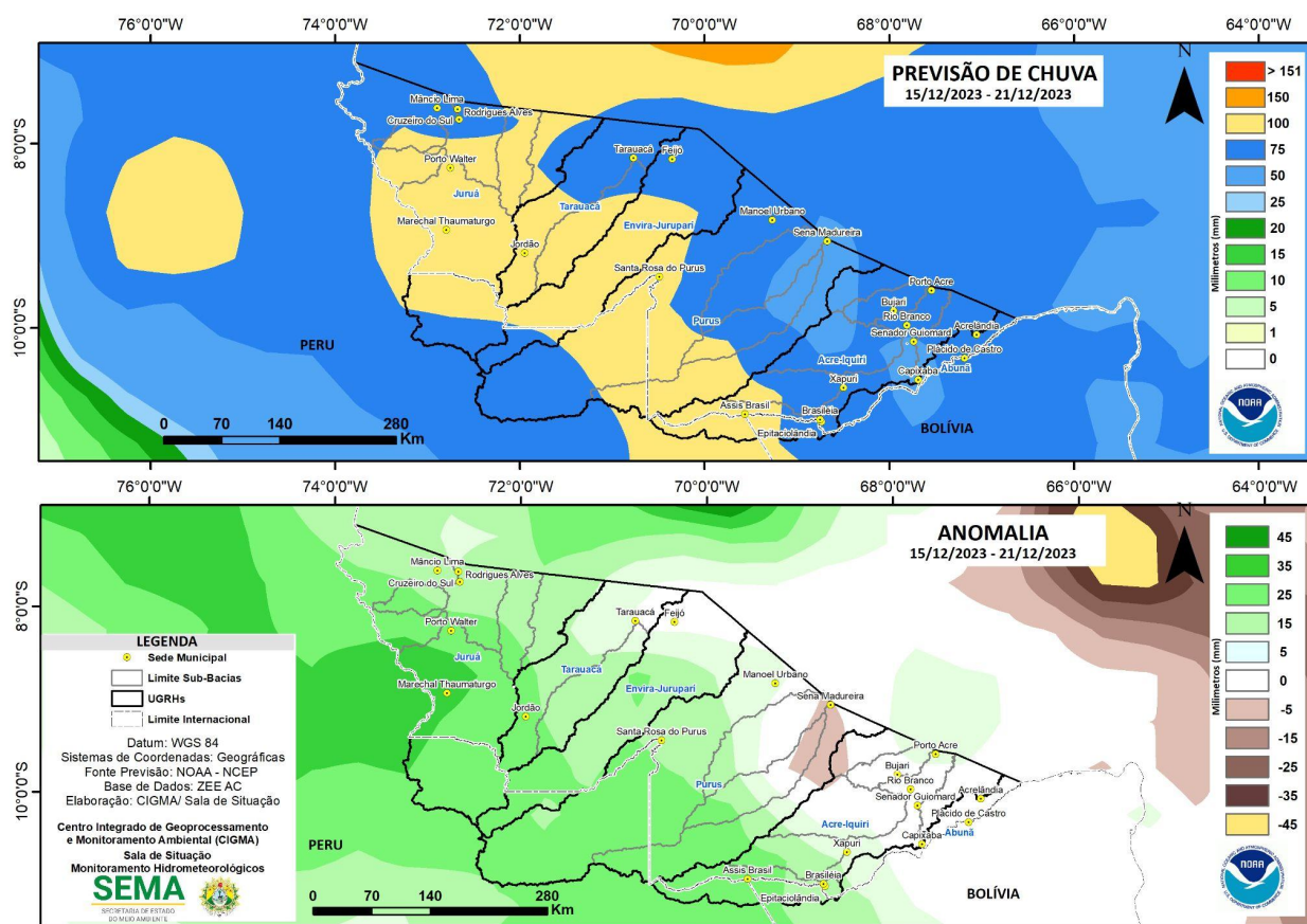
Figura 2: Prognóstico NCEP-GFS
