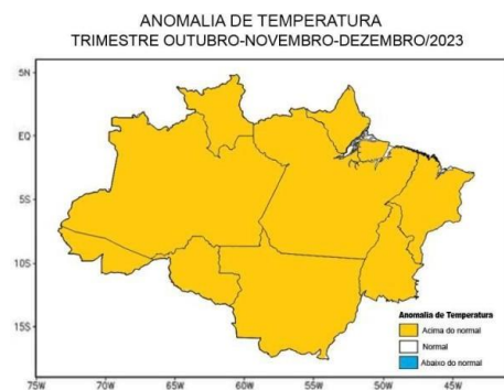
Figura 03 - Prognóstico de anomalias de temperatura para o trimestre Outubro-Novembro-Dezembro/2023.
