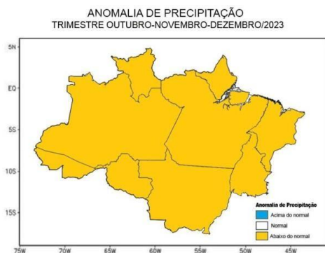
Figura 02 - Prognóstico de anomalias de precipitação para o trimestre Outubro-Novembro-Dezembro/2023.
