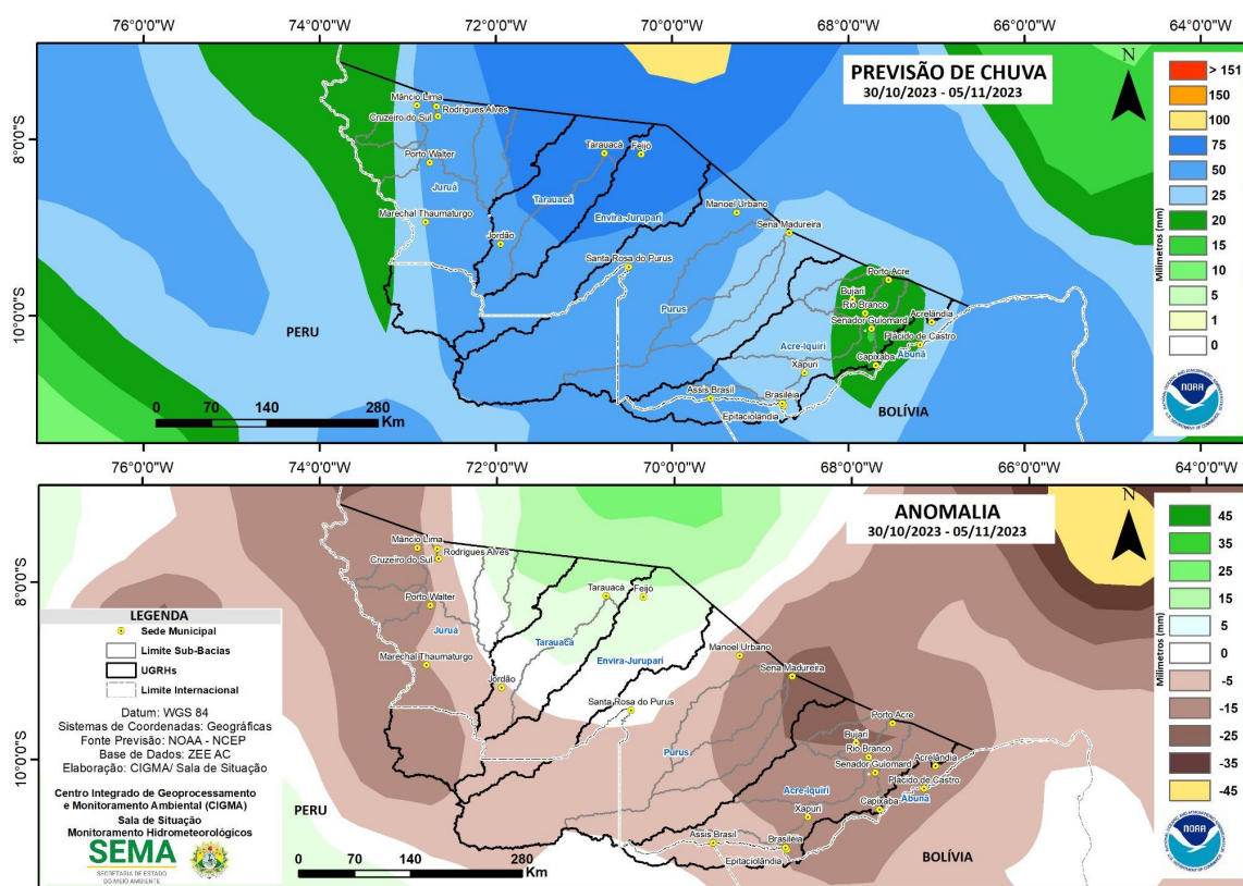
Figura 2: Prognóstico NCEP-GFS
