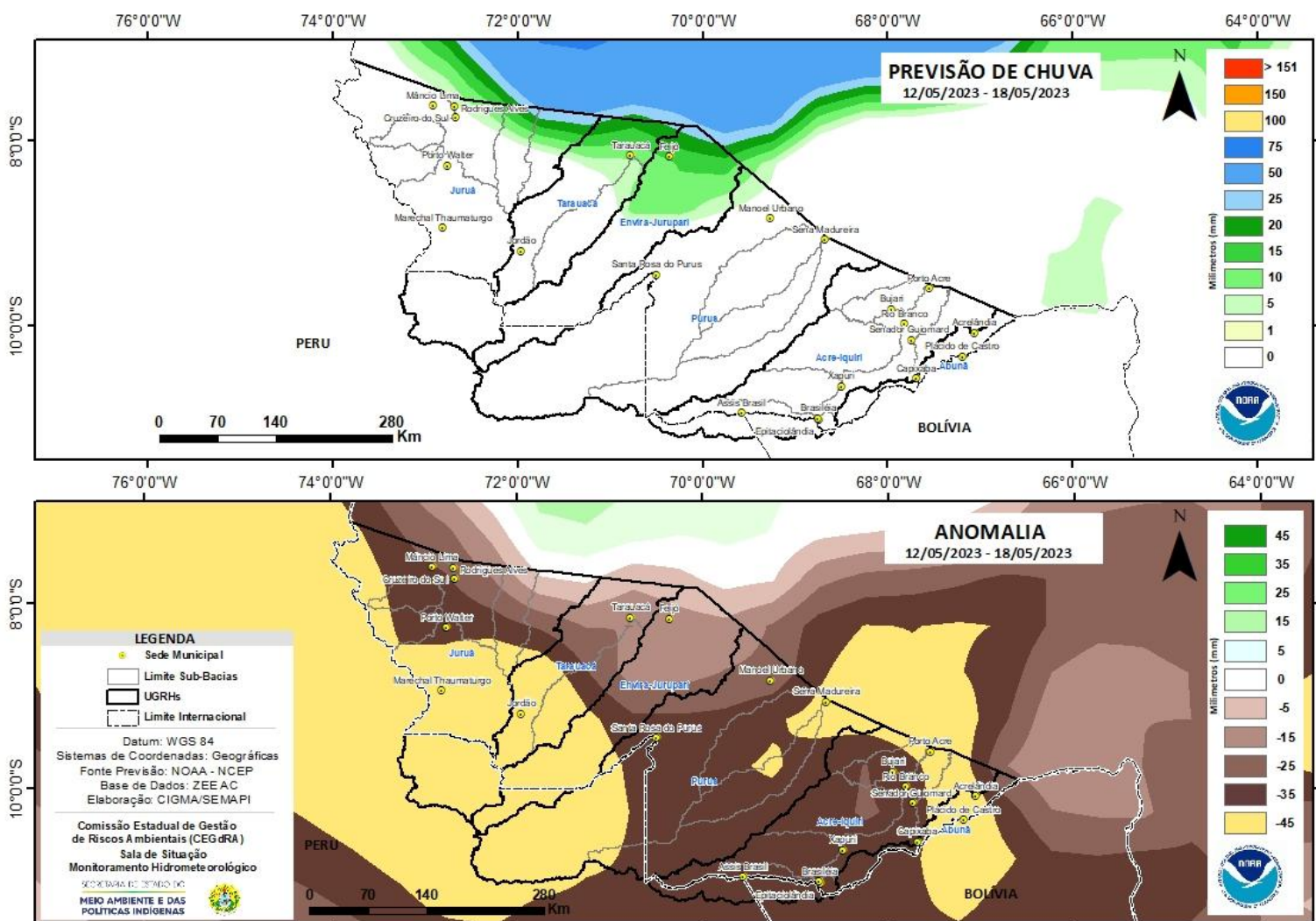
Figura 2: Prognóstico NCEP-GFS/USA.
