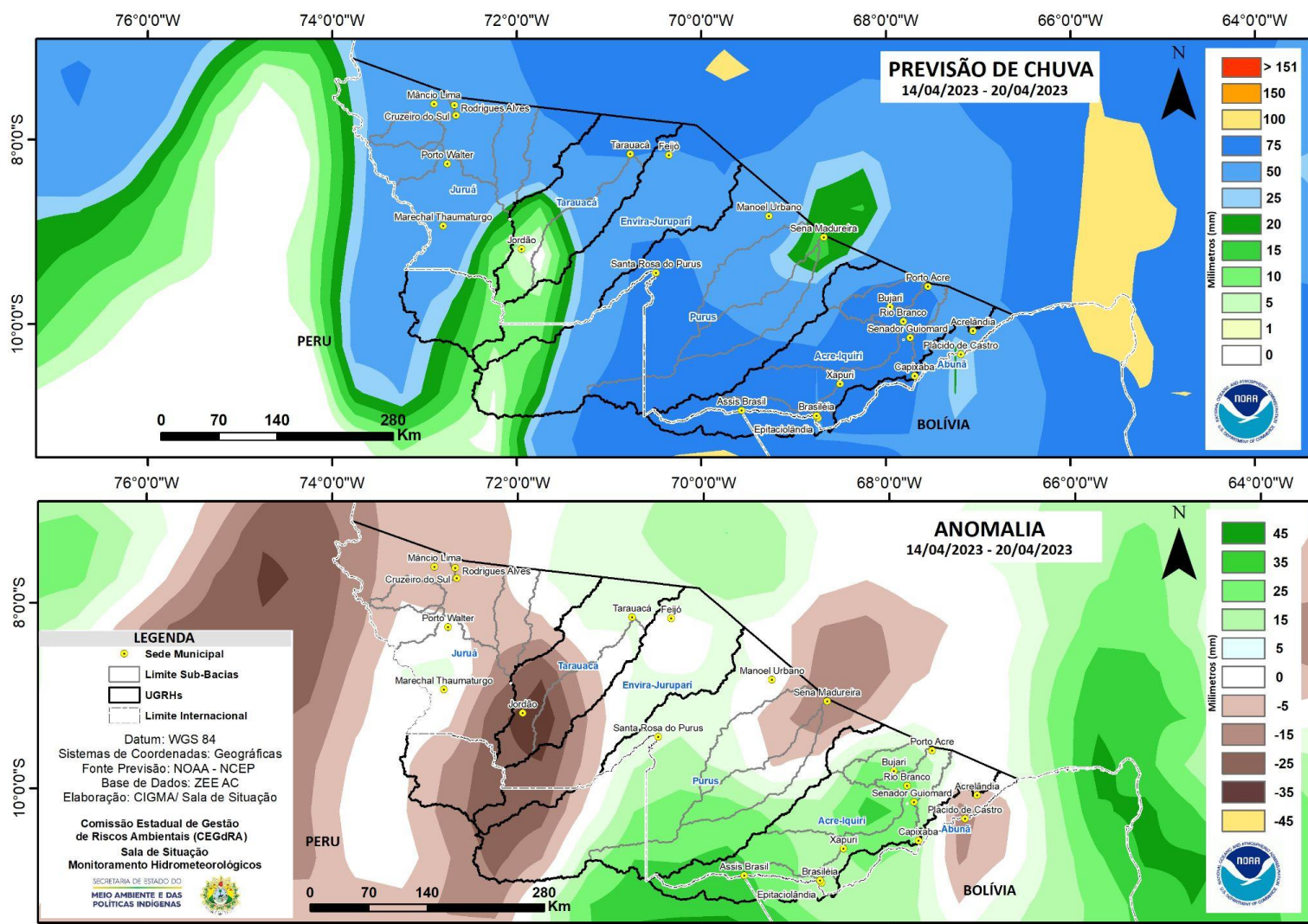
Figura 2: Prognóstico NCEP-GFS/USA.
