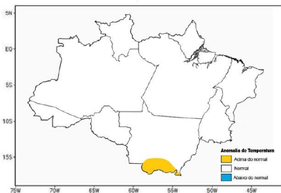
Figura 03 - Prognóstico de anomalias de temperatura para o trimestre Março-Abril-Maio/2023.
