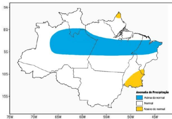
Figura 02 - Prognóstico de anomalias de precipitação para o trimestre Março-Abril-Maio/2023.
