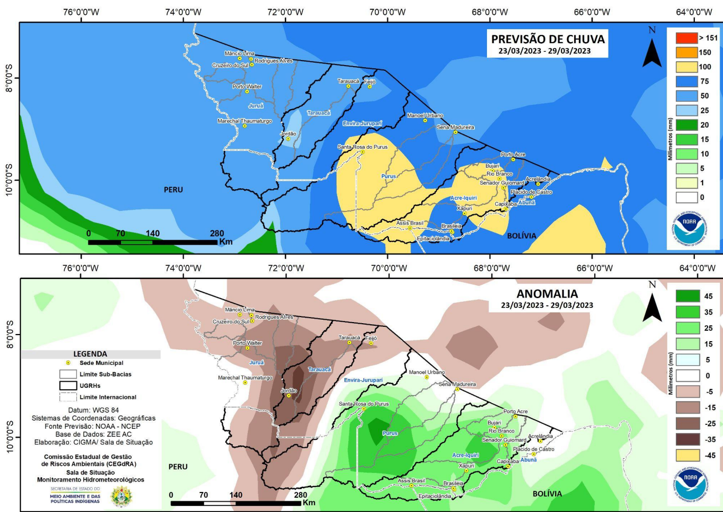
Figura 2: Prognóstico NCEP-GFS/USA.
